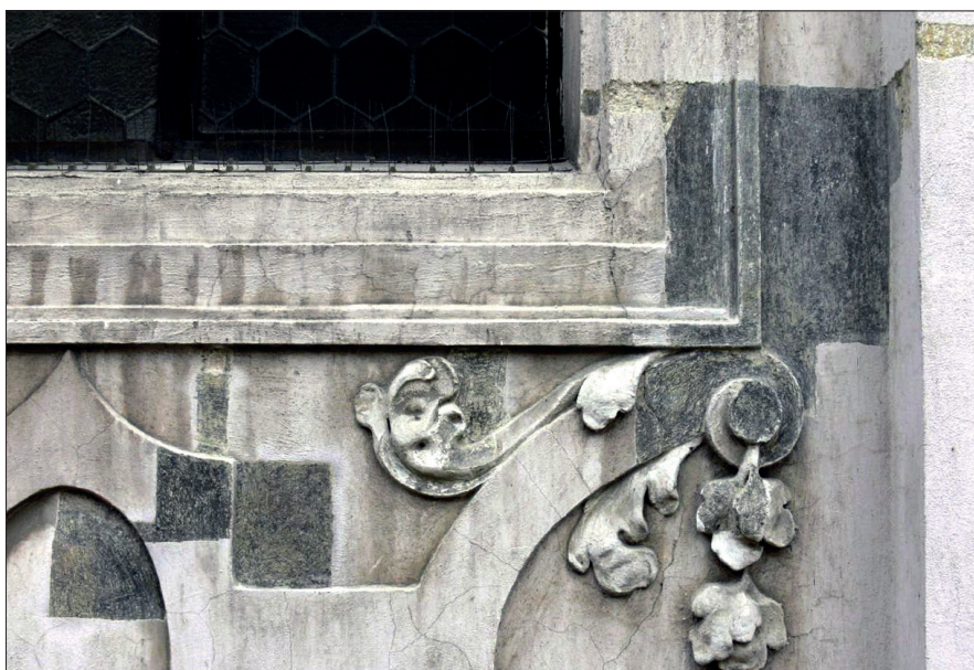
Obr. 26. Sondážně odhalený povrch omítky s výrazně šedou barevností. Kompaktnost a homogenita povrchu i jednodušnost šedého zbarvení v praxi může vést k domněnce, že se jedná o nátěr černé či tmavě šedé barevnosti. Jak dokládá obrázek 27, stratigrafický průzkum v těchto případech obvykle dobře odliší nátěr od znečištění.
