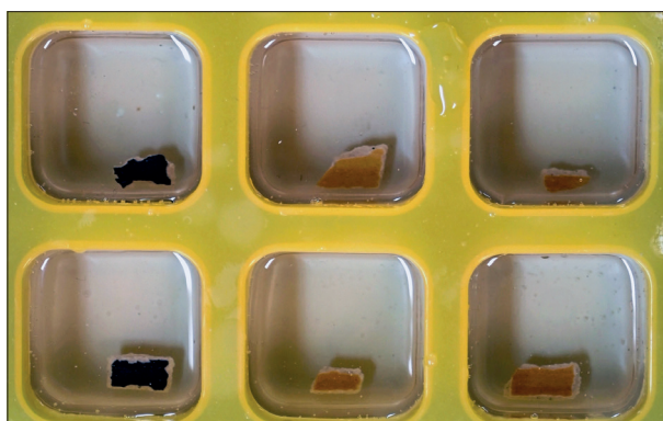
Obr. 11. Forma se vzorky z obr. 10 po zalití a vytvorení pryskyřice. Z porovnání snímků před a po zalití je dobře patrné prosycení nátěrů pryskyřicí.
